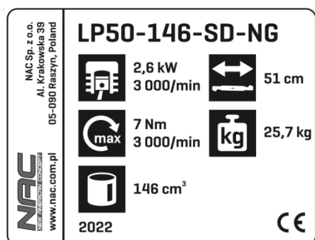
Typový štítok
