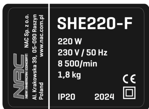
Typový štítok
